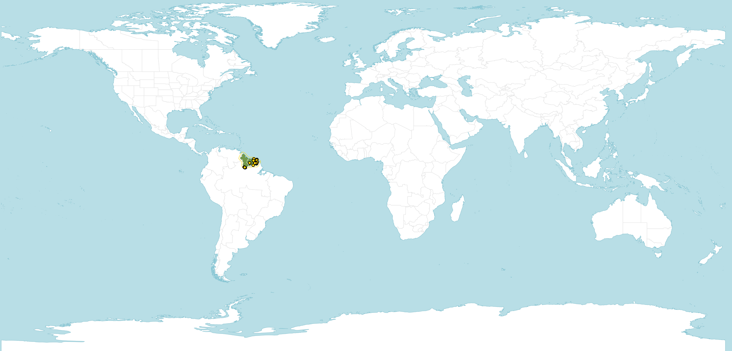
226. Eugenia tetramera
